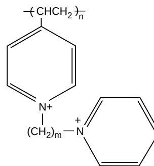
(d) Pyridinium
